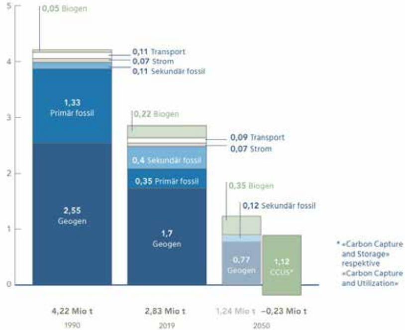
CEMSUISSE 2021, Roadmap 2050
